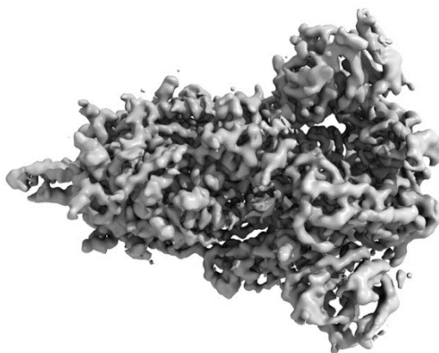
Struktura Cryo-EM białek „spike” SARS-CoV-2 na nienaruszonych wirionach (z bazy Electron Microscopy Data Bank EMD-11497)
